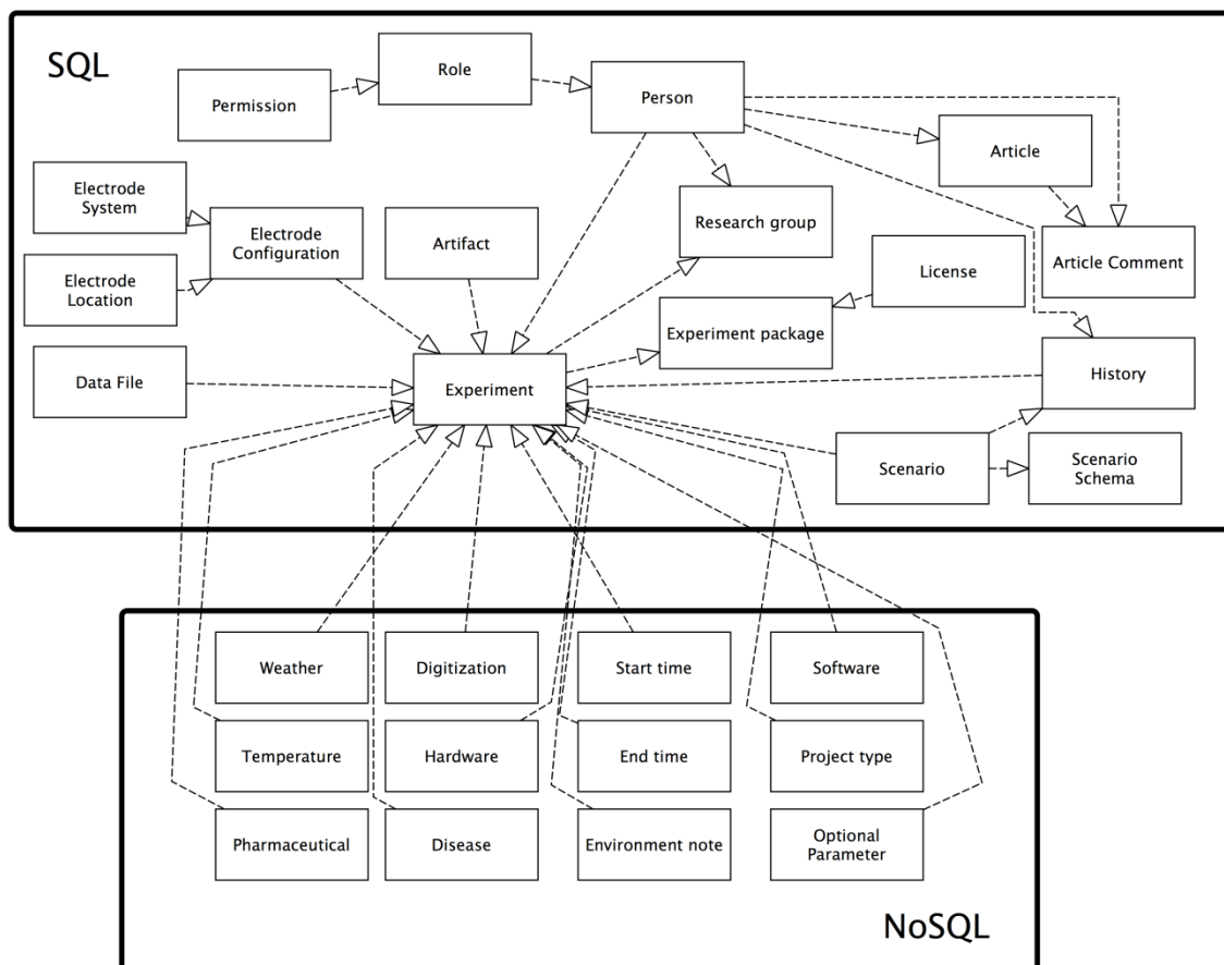
Obrázek 3: Vymezení dat SQL vs. NoSQL
