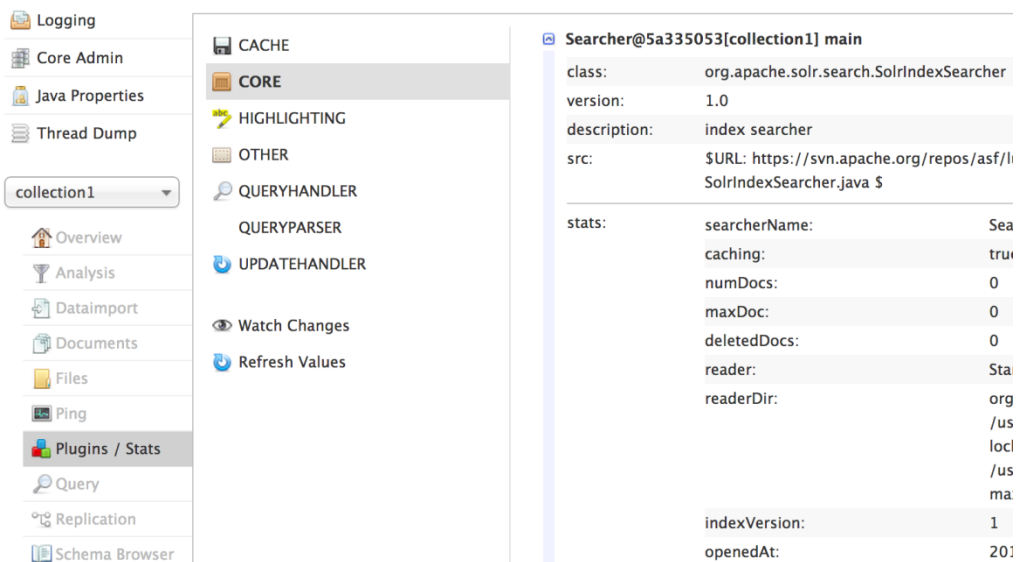
Obrázek 6: Solr monitoring
