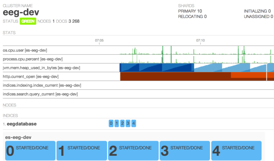
Obrázek 5: Elasticsearch monitoring
