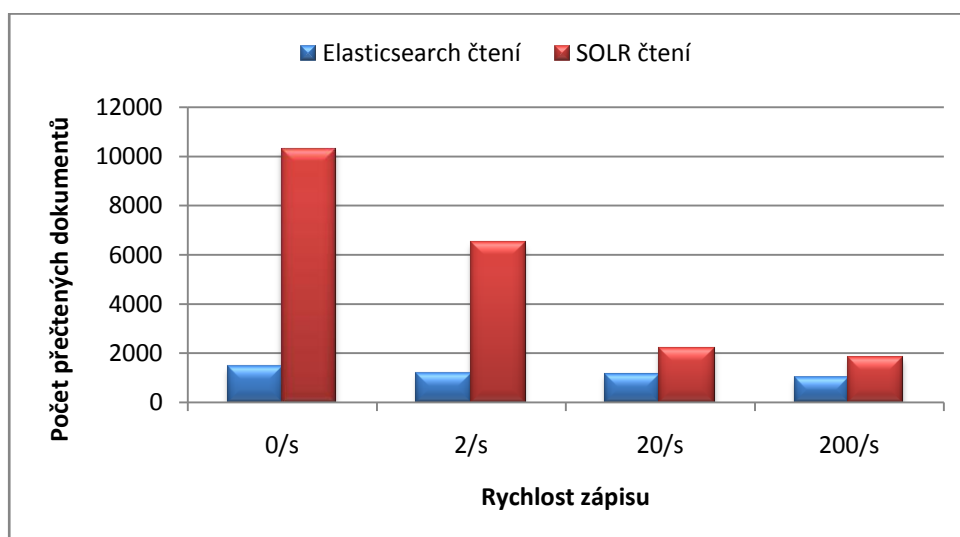
Obrázek 7: Srovnání výkonu Elasticsearch vs. SOLR
