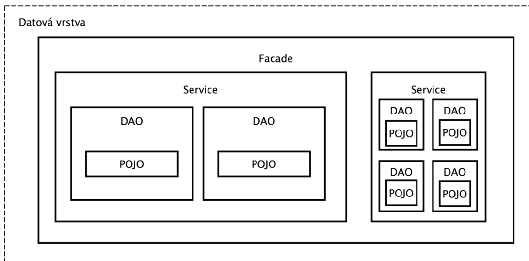
Obrázek 2: Architektura datové vrstvy
