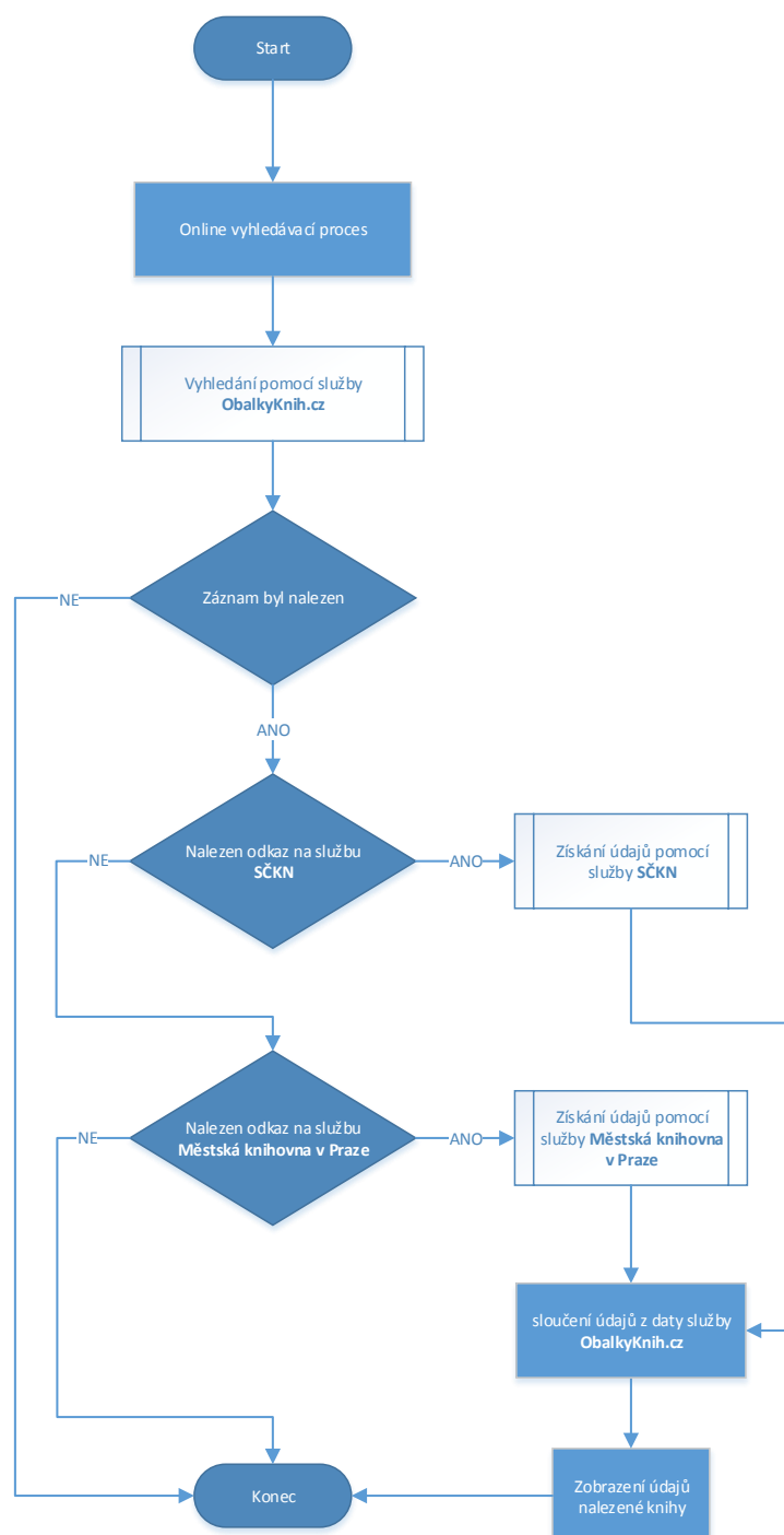
Obrázek 5.3: Vývojový diagram vyhledávače
