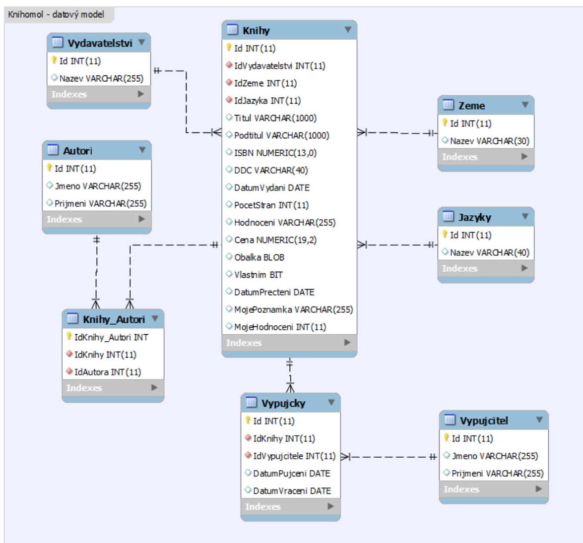
Obrázek 5.1: Databázový model navržený v aplikaci MySQL WorkBench
