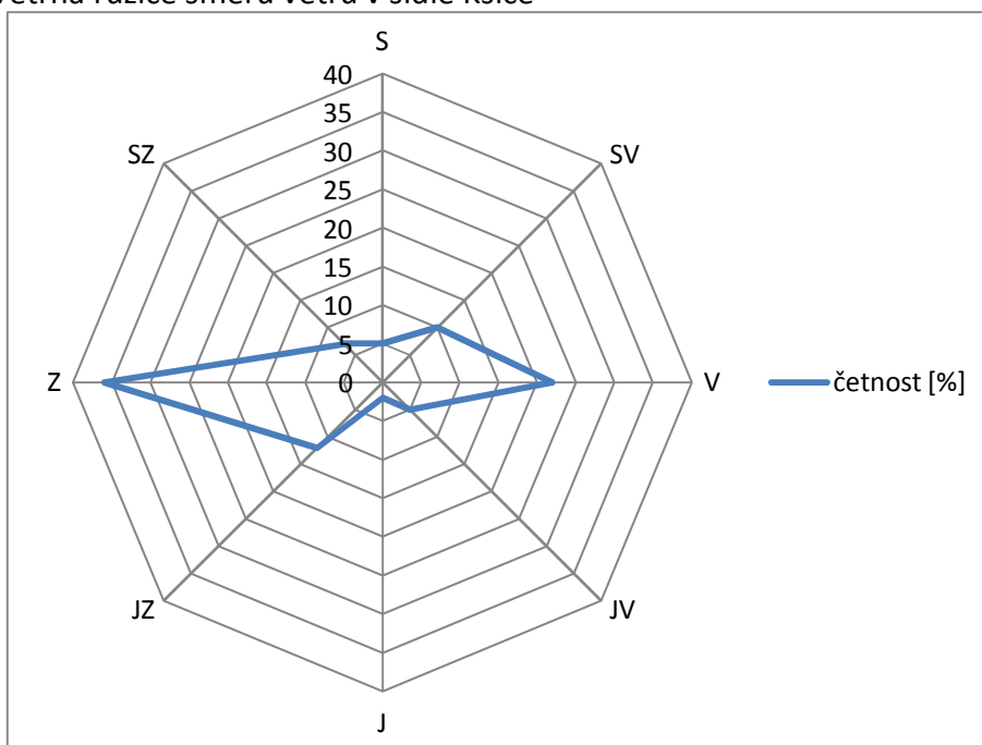
Graf č. 2 Větrná růžice směru větru v sídle Kšice
