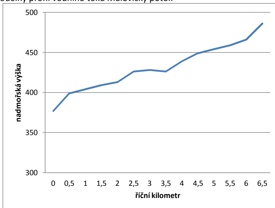
Graf č. 3 Podélný profil vodního toku Malovický potok
