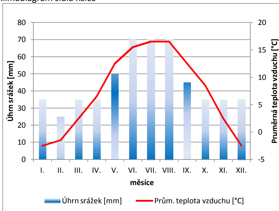
Graf č. 1 Klimadiagram sídla Kšice
