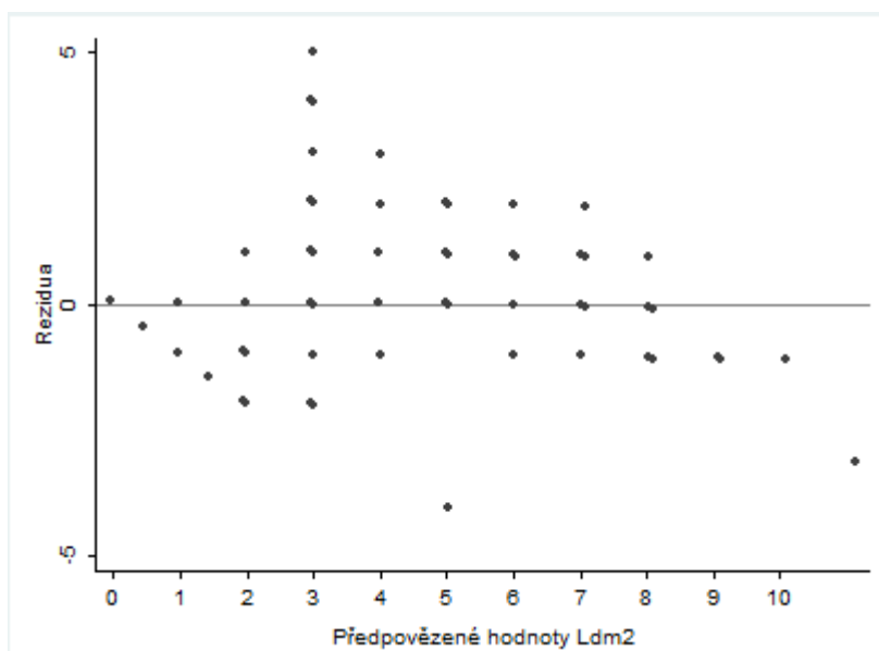
Graf IV.: Rozdíly v předpovězených a naměřených hodnotách u Ldm2.
