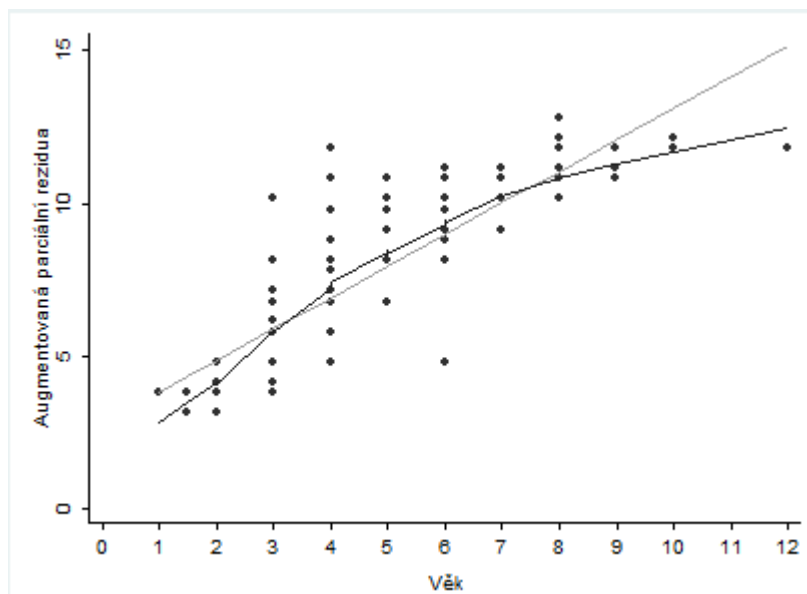
Graf 5.: Testování linearitu vztahu predikční proměnné pro Ldm2. Tmavě šedá představuje linearitu testované proměnné, světle šedě je vyznačen ideální stav.
