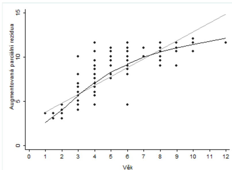
Graf 3.: Testování linearity vztahu predikční proměnné pro Rdm2. Tmavě šedá představuje linearitu testované proměnné, světle šedě je vyznačen ideální stav.
