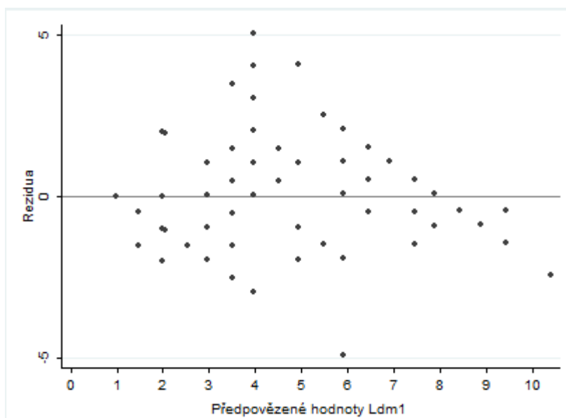
Graf III.: Rozdíly v předpovězených a naměřených hodnotách u Ldm1.
