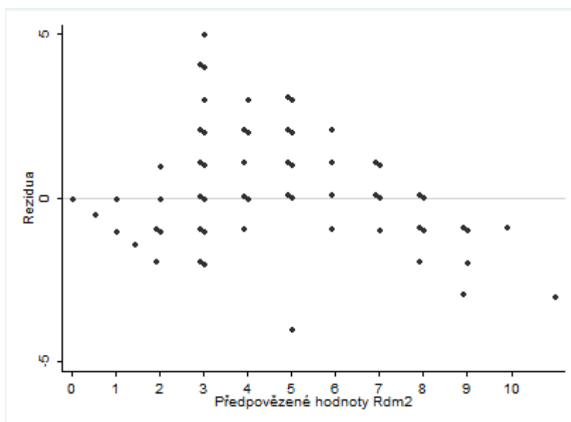
Graf II.: Rozdíl mezi předpovězenými a naměřenými hodnotami u Rdm2.
