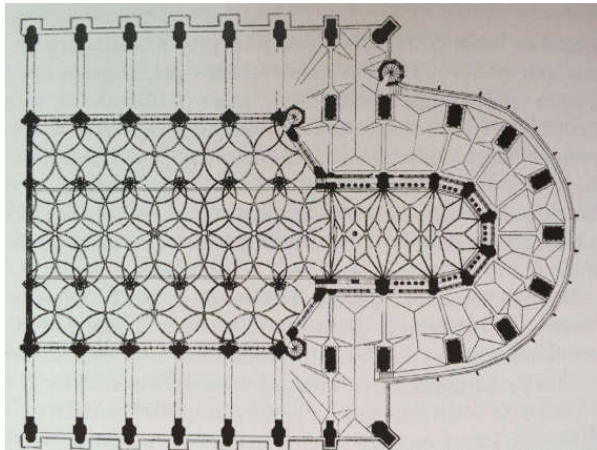
Příloha č. 2. Kostel sv. Barbory v Kutné Hoře, půdorys. Dle Braniš 1893. Kopie z knihy: KALINA, Pavel. Benedikt Ried a počátky záalpské renesance . [Česko] : P. Kalina, 2009, s. 164.
