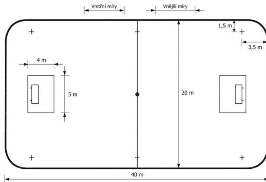
Obrázek č. 4: Nákres hřiště s rozměry (zdroj: http://www.tepsport.wz.cz ).
