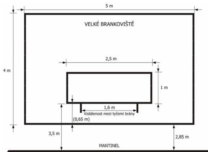
Obrázek č. 5: Nákres brankoviště s rozměry (zdroj: http://www.tepsport.wz.cz ).
