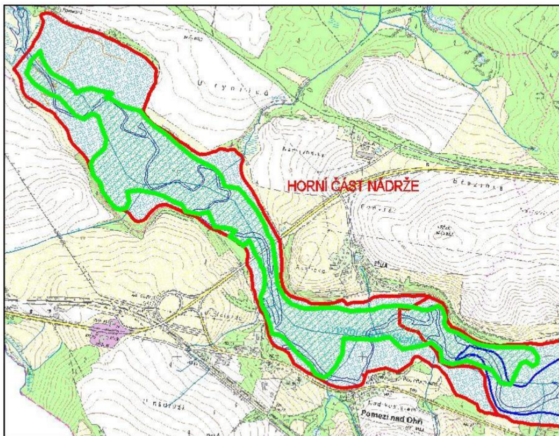
Obrázek č. 13: Oblast rizikového sedimentu ve VD Skalka
