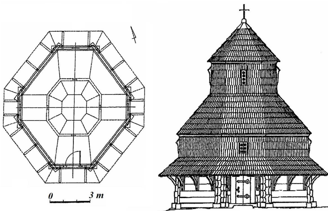
Obr. 21 Rekonstrukce dřevěného kostela na lokalitě Voskresens'ke (LUKOMSKY 2001, 295)
