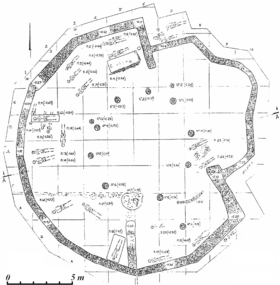
Obr. 20 Půdorys Olešivské rotundy (TOMENČUK 2008, 247)
