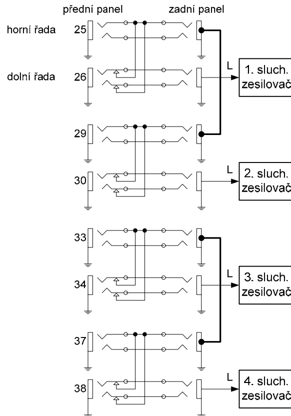
Obr. 14: Zapojení sluchákových zesilovačů na Patch-Bay přepojovači
