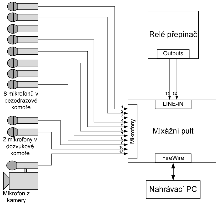
Obr. 10: Připojené mikrofonní a linkové vstupy mixážního pultu
