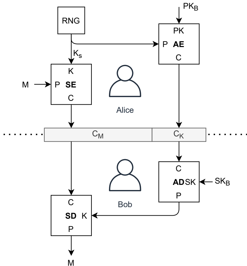
Obrázek 3.1: Proces šifrování zprávy M v OpenPGP, odeslán je šifrový text zprávy C_M spolu s šifrovaným relačním klíčem C_K . Význam použité bloků je: Symetric encryption (SE) – symetrická šifra, vstupem je klíč K a otevřený text P , výstupem je šifrový text C . Symetric decryption (SD) – šifrový text C symetricky dešifruje. Asymmetric encryption (AE) – asymetricky šifruje Bobovým veřejným klíčem PK_B . Asymmetric decryption (AD) – dešifruje asymetrickou šifru Bobovým privátním klíčem SK_B . Random number generator (RNG) – zdroj náhodných dat.
