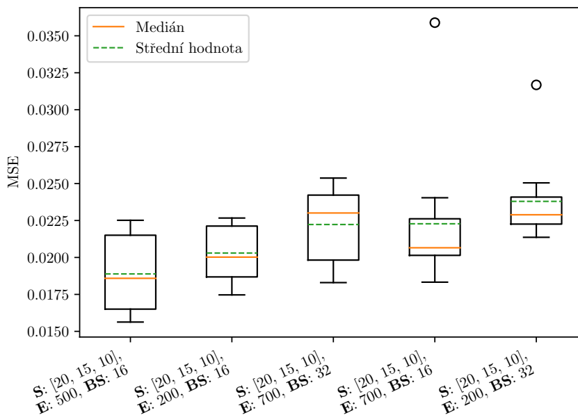
OBRÁZEK 7.3: Boxplot realizací prvních 5 nejlepších modelů dopředné neuronové sítě (FFNN)
