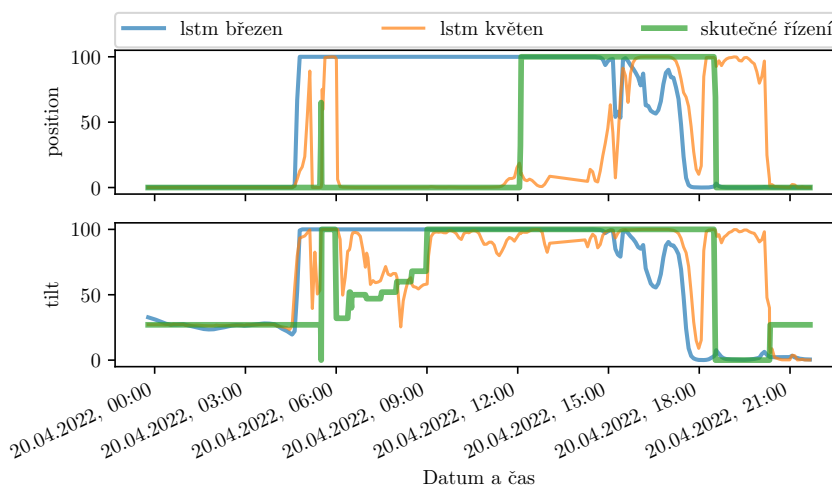
OBRÁZEK 7.11: Porovnání predikce 2 modelů LSTM a skutečného řízení na datech z 20. dubna 2022
