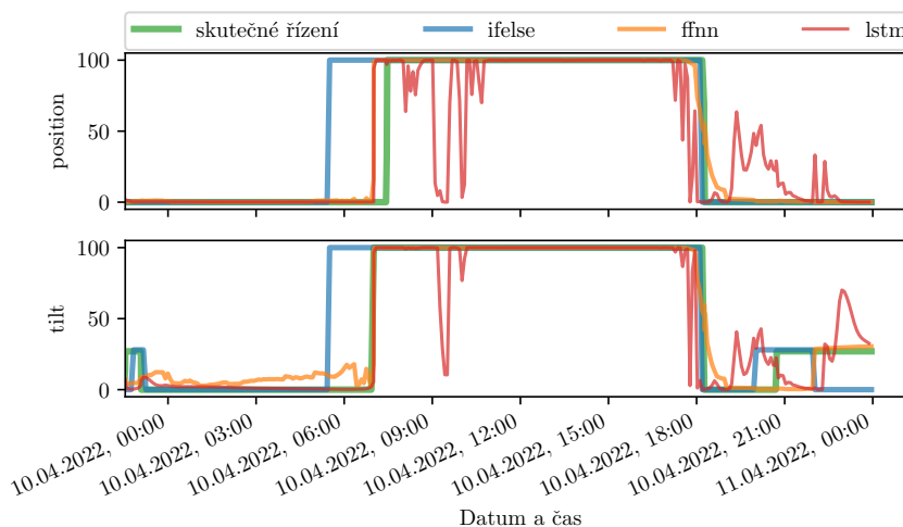
OBRÁZEK 7.9: Porovnání predikce 3 regresorů a skutečného řízení na datech z 10. dubna 2022
