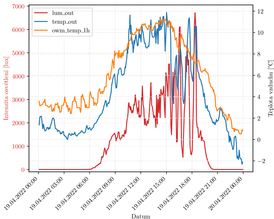
OBRÁZEK 7.1: Graf sesbíraných hodnot 3 vybraných příznakových veličin z celkových 15. Zobrazena je pouze část dat ze dne 19. dubna 2022
