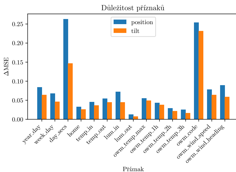
OBRÁZEK 7.8: důležitostst příznaků metodou nulování v regresoru založeném na rekurentní neuronové síti v úloze automatického ovládání žaluzie.
