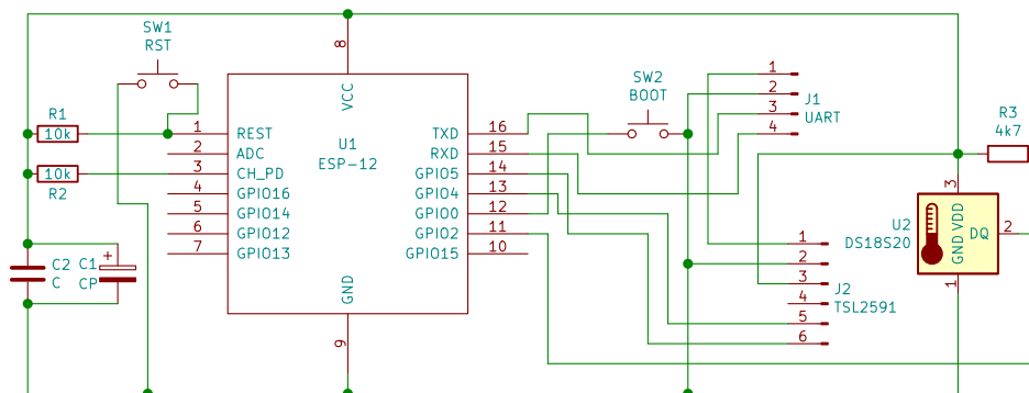
OBRAZEK 3.2: Schéma zapojení zařízení, která měří intenzitu osvětlení pomocí senzoru TSL2591 a teplotu vzduchu pomocí senzoru DS18B20. Hodnoty se přenášejí přes WiFi.
