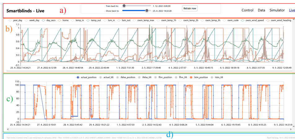
OBRÁZEK 6.6: Stránka Live v grafickém uživatelském rozhraní systému pro automatické ovládání žaluzií s vyznačenými částmi pomocí barevných obdélníků a) – d)
