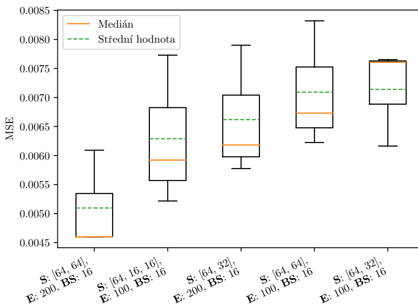
OBRÁZEK 7.4: Boxplot realizací prvních 5 nejlepších modelů rekurentní neuronové sítě LSTM
