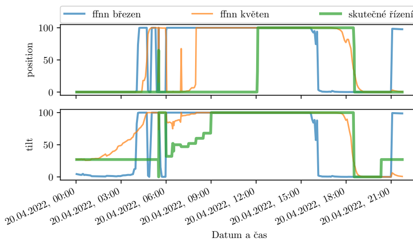
OBRÁZEK 7.10: Porovnání predikce 2 modelů dopředné neuronové sítě a skutečného řízení na datech z 20. dubna 2022
