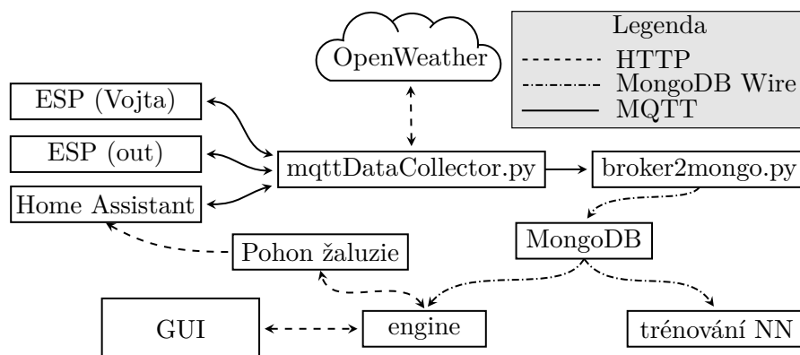
OBRÁZEK 4.1: Schéma komunikace komponent systému automatického řízení žaluzií, tok dat mezi nimi a komunikační protokoly.
