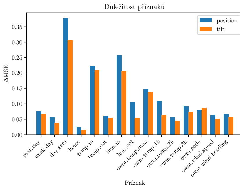
OBRÁZEK 7.7: důležitostst příznaků metodou nulování v regresoru založeném na dopředné neuronové síti v úloze automatického ovládání žaluzie.
