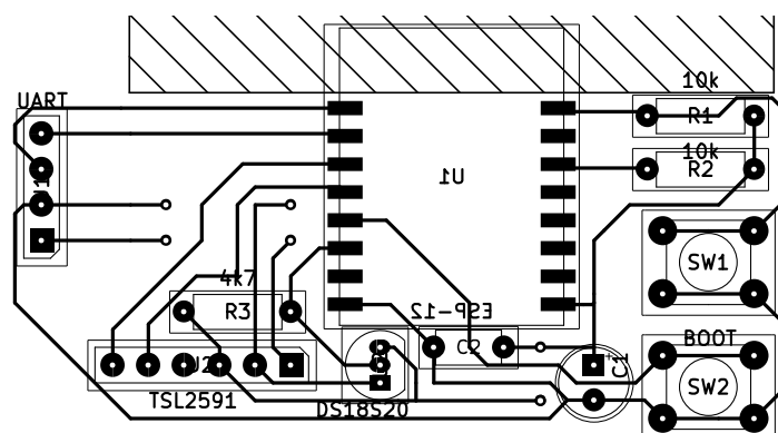
OBRAZEK 3.3: Návrh desky plošných spojů zařízení, která měří intenzitu osvětlení pomocí senzoru TSL2591 a teplotu vzduchu pomocí senzoru DS18B20. Hodnoty se přenášejí přes WiFi. Šrafovaná oblast je ochranná zóna antény.
