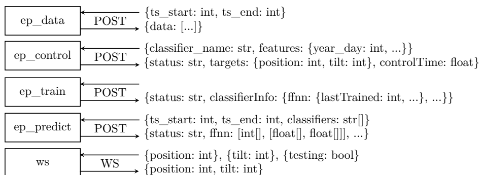
OBRÁZEK 4.2: Schéma endpointů backendu systému pro automatické ovládání žaluzií a datové struktury přenášené v těle jednotlivých požadavků a odpovědí včetně metody. V posledním případě se jedná o protokol WebSockets.
