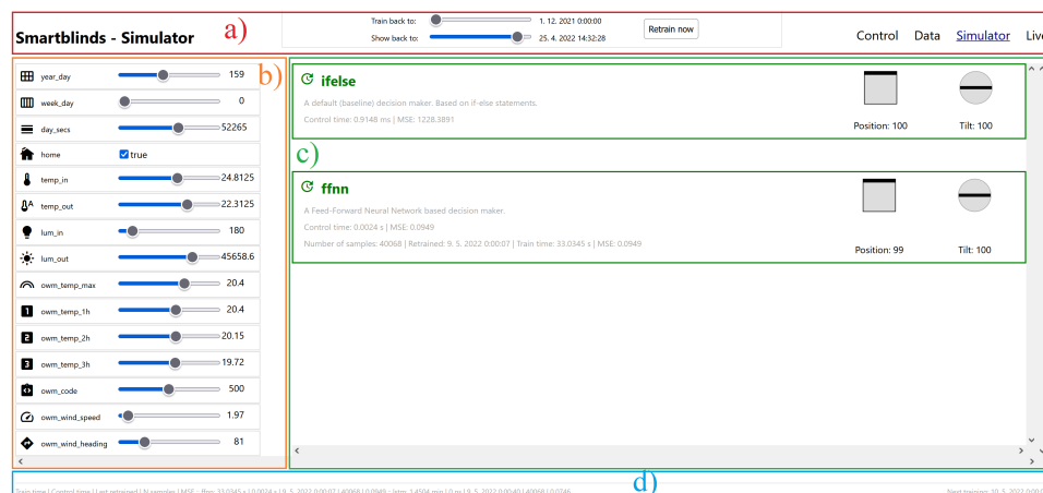
OBRÁZEK 6.3: Stránka Simulator v grafickém uživatelském rozhraní systému pro automatické ovládání žaluzií s vyznačenými částmi pomocí barevných obdélníků a) – d)
