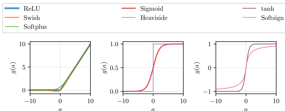
OBRÁZEK 1.1: Grafy vybraných aktivačních funkcí
