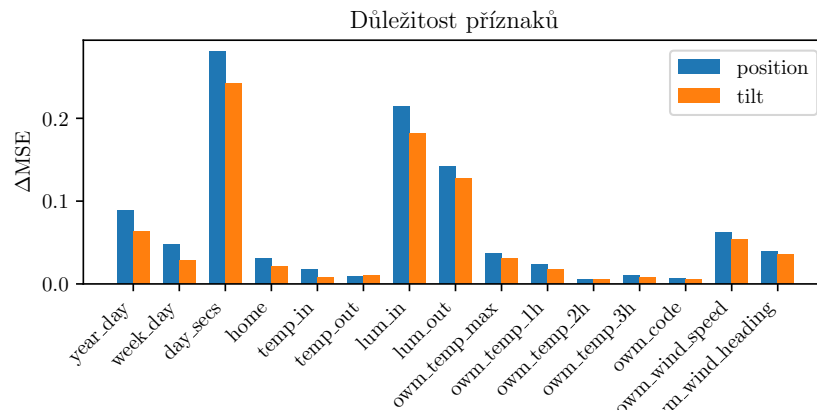
OBRÁZEK 7.5: Permutační důležitostst příznaků v regresoru založeném na dopředné neuronové síti v úloze automatického ovládání žaluzie.
