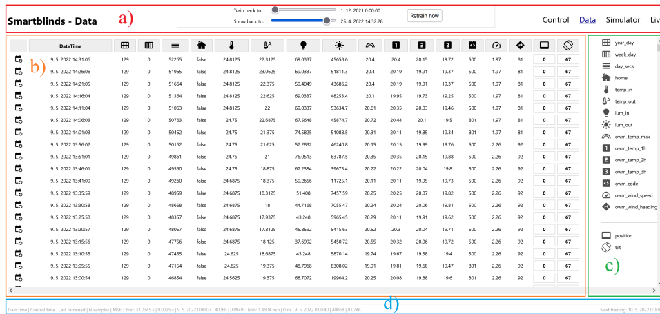
OBRÁZEK 6.2: Stránka Data v grafickém uživatelském rozhraní systému pro automatické ovládání žaluzií s vyznačenými částmi pomocí barevných obdélníků a) – d)
