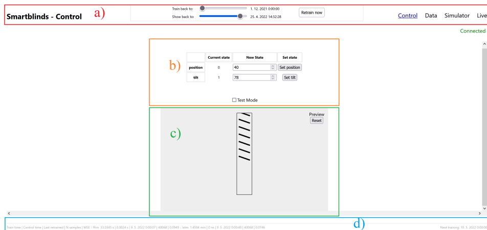
OBRÁZEK 6.5: Stránka Control v grafickém uživatelském rozhraní systému pro automatické ovládání žaluzií s vyznačenými částmi pomocí barevných obdélníků a) – d)
