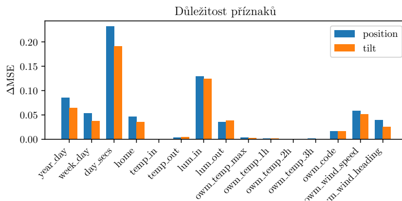
OBRÁZEK 7.6: Permutační důležitostst příznaků v regresoru založeném na rekurentní neuronové síti v úloze automatického ovládání žaluzie.
