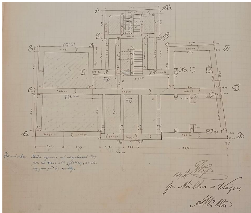
Obrázek 25: Půdorys zdi staré školní budovy
